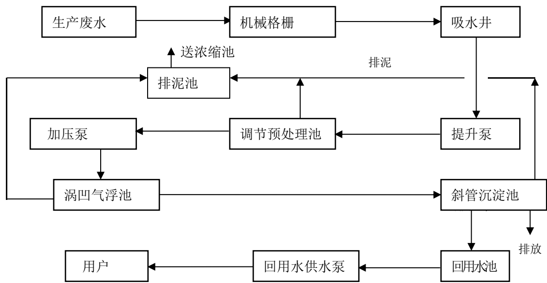
图 2.5—1 现有生产废水预处理系统工艺流程图
