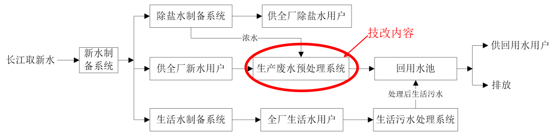
图 2.3—1 重钢水处理现状系统流程框图
