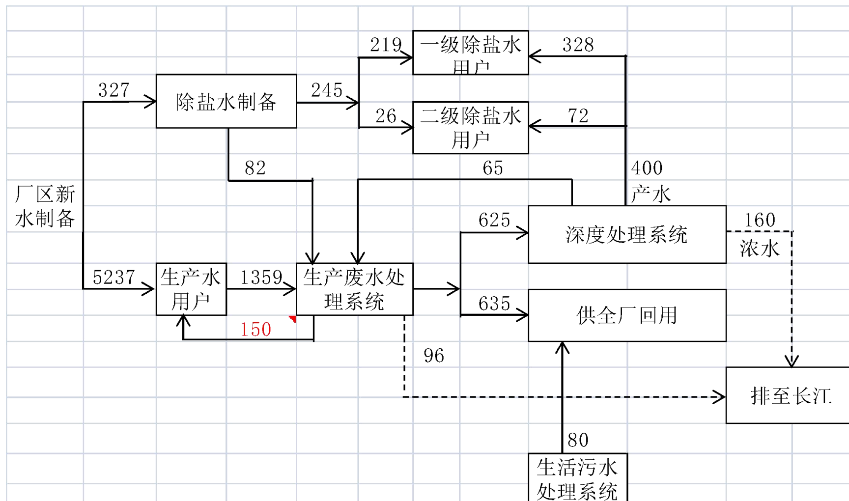
图 3.2-2 扩建后重钢废水处理系统水平衡图 \text{m}^3/\text{h}
