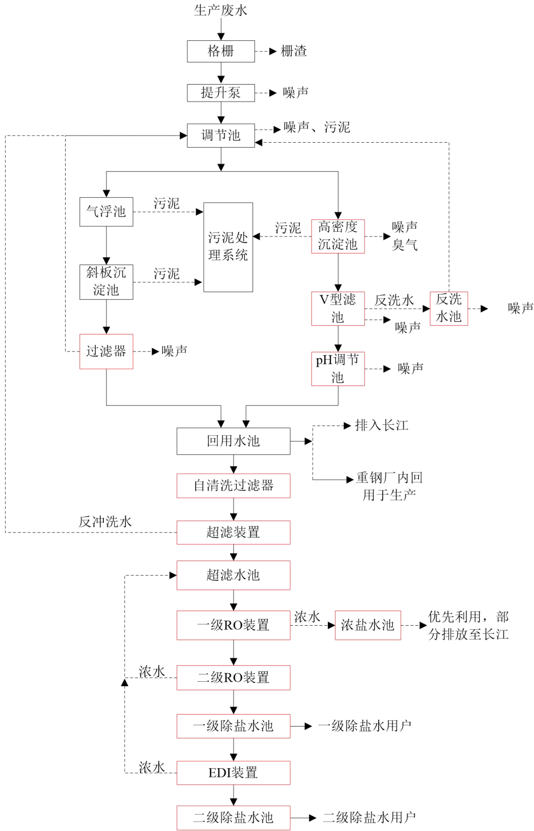
图 3.2—2 工艺流程及产污环节图
