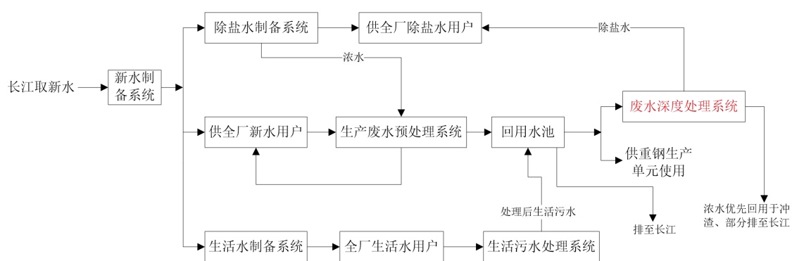
图 3.2—1 重钢全厂水处理系统流程图
