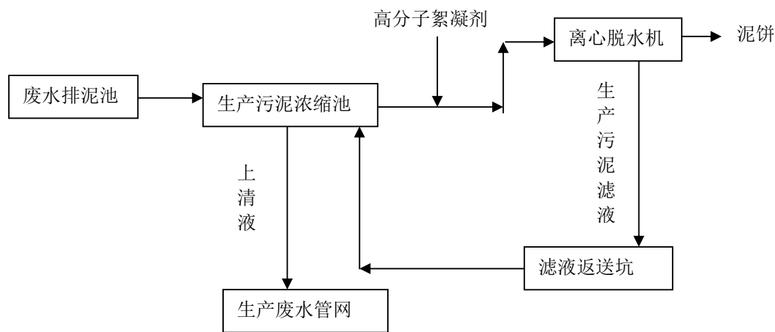
图 2.5—2 现有污泥处理系统工艺流程图
