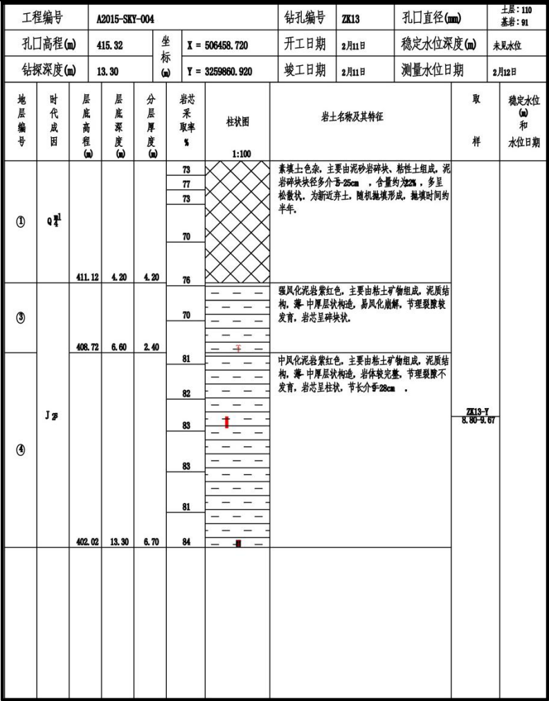
图 4.1—1 建设场地典型钻孔柱状图
