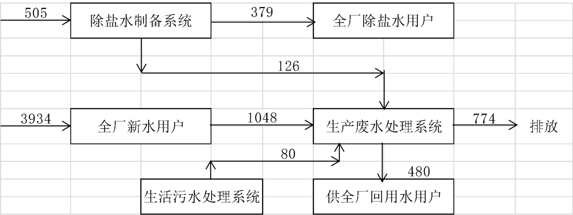
图 2.6-1 重钢现状水平衡图 m³/h
